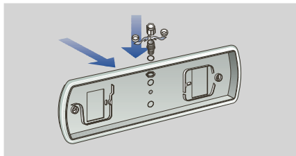
Införingspunkter för kablage.
