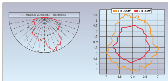
Ljusflöde vid montagehöjd 3 m från golv, ljuskälla PL 24W.
